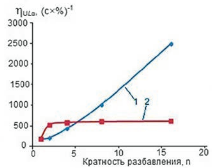
Рис. 5. Зависимость дифференциальной чувствительности для аналитической линии UL\alpha при разбавлении кориумного материала тетраборатом лития 1 и оксидом цинка 2.
