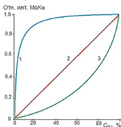
Рис. 1. Зависимость относительной интенсивности аналитической линии MoK \alpha в легком наполнителе 1, в нейтральном наполнителе 2 и в тяжелом наполнителе 3.
