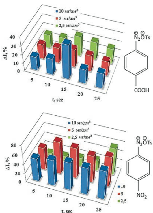
Рис. 5. Влияние времени модификации УСЭ COOH-C 6 H 4 N 2 + TsO - (а) и NO 2 -C 6 H 4 N 2 + TsO - (б) на токи окисления 50 моль/дм 3 кофеина.
