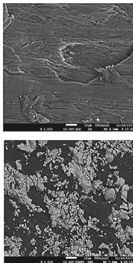
Рис. 6. Морфология поверхности УСЭ (а) и УСЭ, модифицированного NO 2 -C 6 H 4 N 2 + TsO - по данным сканирующей электронной микроскопии. Концентрация модификатора 5 мг/л, время модификации 10 с.
