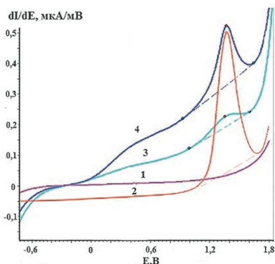
Рис. 3. Дифференциальные анодные ВА первого порядка 50 моль/дм 3 кофеина на УСЭ (кривая 2), электрохимически модифицированных COOH-C_6H_4N_2^+TsO^- -УСЭ (кривая 3) и NO_2-C_6H_4N_2^+TsO^- -УСЭ (кривая 4) на фоне 0.05 М H_2SO_4 (кривая 1). \nu = 80 мВ/с.
