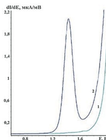
Рис. 4. Дифференциальные анодные ВА первого порядка 50 моль/дм 3 кофеина на УСЭ (кривая 2), электрохимически модифицированных COOH-C_6H_4N_2^+TsO^- -УСЭ (а) и NO_2-C_6H_4N_2^+TsO^- -УСЭ (б) на фоне 0.05 М H_2SO_4 (кривая 1). \nu = 80 мВ/с.
