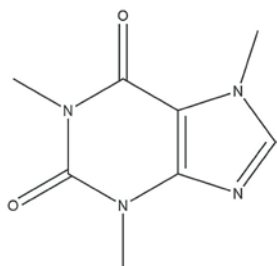
Рис. 1. Структурная формула кофеина (3,7-дигидро-1,3,7-триметил-1H-пурин-2,6-дион).
