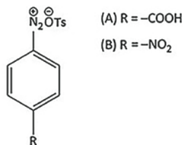
Рис. 2. Структурная формула тозилатных солей арендиазония.
