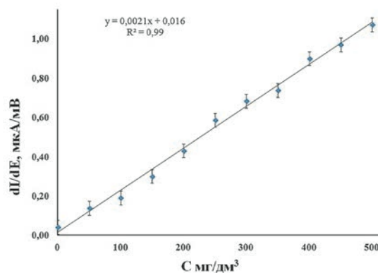
Рис. 8. Градуировочный график для определения кофеина в модельных растворах.
