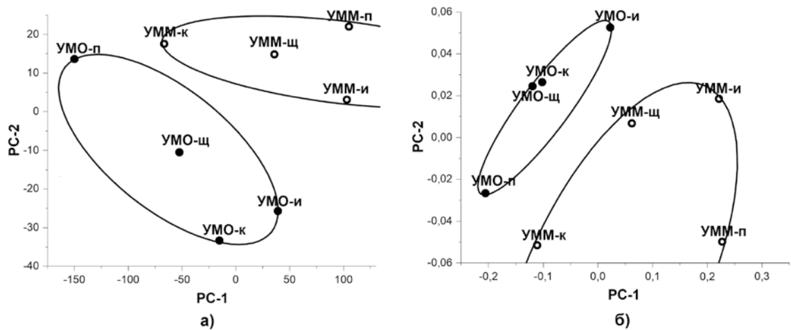
Рис. 3. График счетов, построенный с использованием всех физических показателей (а), и с использованием двух показателей - A^{daf} и S_{БЭТ} (б) Fig. 3. Scores graph with use of all physical characteristics and with the use of A^{daf} and S_{БЭТ} only
