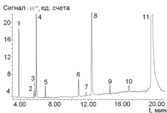
Рис. 1. Хроматограмма концентрата примесей, полученная с использованием колонки GS-GasPro. 1 – N 2 , Ar, O 2 , 2 – C 2 H 6 , 3 – N 2 O, 4 – CO 2 , 5 – C 2 H 4 , 6 – C 2 H 2 , COS, 7 – C 3 H 8 , 8 – H 2 S, 9 – C 3 H 6 , 10 – изо -C 4 H 10 , 11 – CS 2 , SO 2
