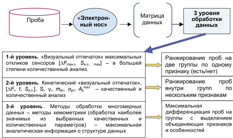
Рис. 2. Общая схема способов анализа результатов для проб различного происхождения
