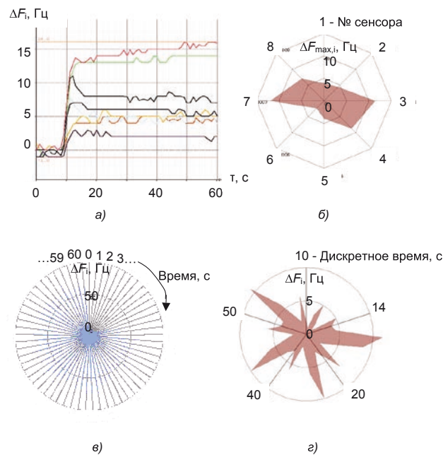
Рис. 1. Визуализация результатов измерения в программном обеспечении для прибора «МАГ-8»: хроночастотограмма (а), «визуальный отпечаток» максимумов (б), полный кинетический «визуальный отпечаток» (в), оптимизированный кинетический «визуальный отпечаток» (г)
