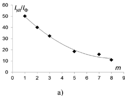
Рис. 4. Зависимость контрастности для MoK \alpha - (а) и CrK \alpha -линий (б) от числа m слоев «фильтра» в излучателе Fig. 4. The dependence of the contrast of the X-ray spectrum for MoK \alpha - (a) and CrK \alpha -lines (b) on the number of m layers of the "filter" in the emitter
