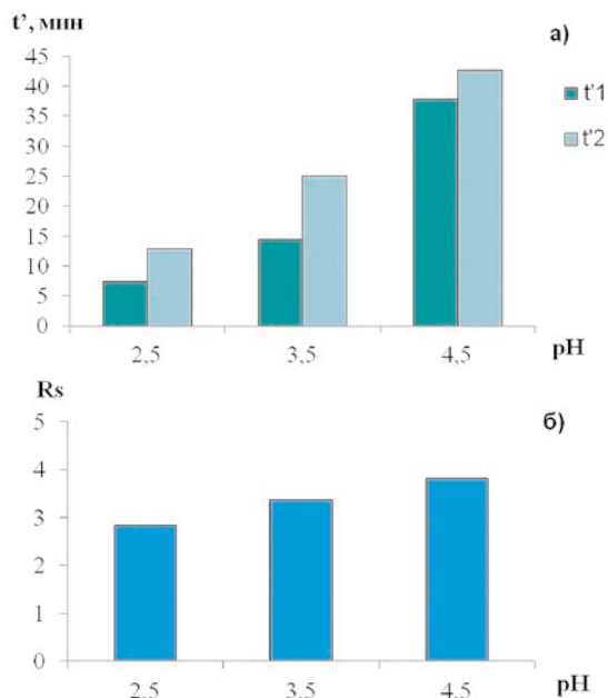
Рис. 4. Влияние pH подвижной фазы на: а – времена удерживания ( t'1 – время удерживания L-изомера, t'2 – время удерживания D-изомера) и б – разрешение пиков энантимеров пеметрекседа. Хроматографическая колонка: Nautilus-E, 250×4 мм. Подвижная фаза: (70 : 30) % об. MeOH : \text{NH}_4\text{H}_2\text{PO}_4 (50 мМ)
