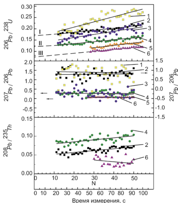
Рис. 4. Типичные зависимости отношений ^{206}\text{Pb}/^{238}\text{U} (A), ^{207}\text{Pb}/^{206}\text{Pb} (Б), ^{208}\text{Pb}/^{232}\text{Th} (B) в цирконах 91500 (1, 2), Mud Tank (3, 4), и GJ-1 (5, 6) от цикла измерения N и времени измерения при диаметре кратера 25 и 50 мкм, соответственно. Показана линейная аппроксимация изотопного отношения ^{206}\text{Pb}/^{238}\text{U} к моменту включения лазера при диаметре кратера 50 мкм для цирконов 91500, Mud Tank и GJ-1 (I, II и III). Изотопные отношения представлены после вычитания сигнала холостого опыта
