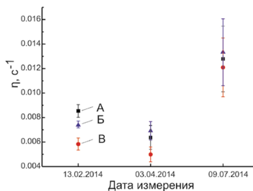
Рис. 7. Величина параметра элементного фракционирования ( \eta , с -1 ) для измеренного изотопного отношения 206 Pb/ 238 U цирконах 91500 (В), GJ (Б) и Mud Tank (А) при идентичных параметрах лазерной установки (50 мкм, 20 Гц, 18-23 Дж/см 2 ) в различные дни измерения: (1) средневзвешенное значение по пяти результатам измерения, (2) средневзвешенное значение по трем результатам измерения, (3) средневзвешенное значение по двум результатам измерения при увеличении времени переключения магнита до 1 с. Погрешность – 2σ
