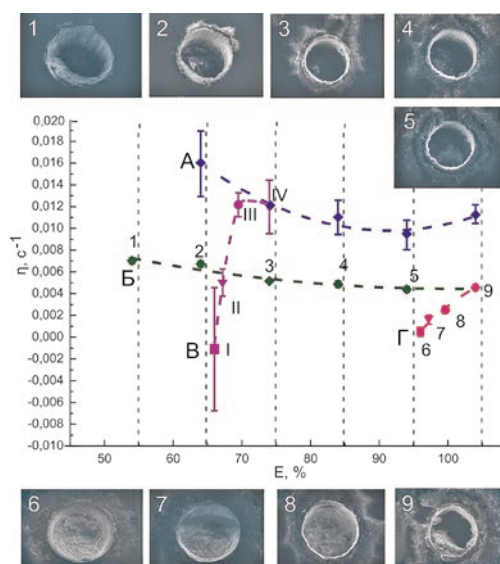
Рис. 5. Величина параметра элементарного фракционирования ( \eta , с -1 ) для измеренного изотопного отношения ^{206}\text{Pb}/^{238}\text{U} в цирконе Mud Tank от энергии лазерного излучения ( E , %) и частоты повторения импульсов (I – 4 Гц; II – 5 Гц; III – 10 Гц; IV – 20 Гц) при: А, В – диаметре кратера 25 мкм; Б, Г – диаметре кратера 50 мкм. 1–9 – внешний вид кратеров после абляции при соответствующих параметрах приставки для ЛА. Пунктирные линии – для наглядности проявления тенденции. Погрешность – 2 \sigma . Внешний вид кратеров при данных параметрах измерения получен на сканирующем электронном микроскопе JSM-6390LV
