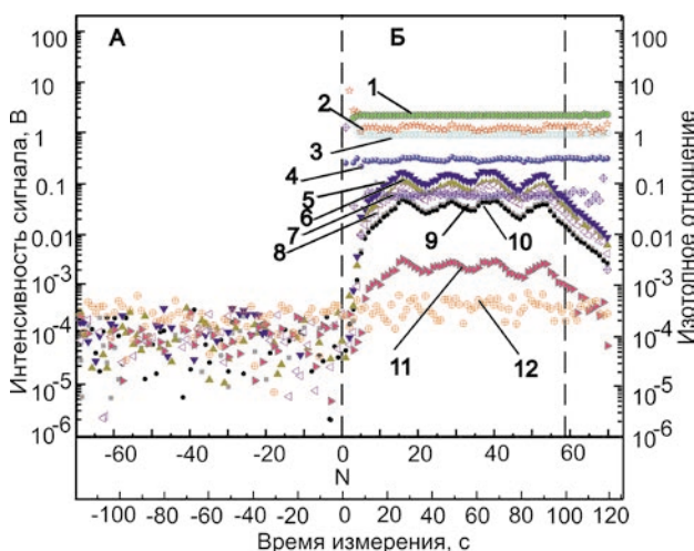
Рис. 2. Типичные сигналы от изотопов ^{202}\text{Hg} (12), ( ^{204}\text{Pb} + ^{204}\text{Hg} ) (11), ^{206}\text{Pb} (9), ^{207}\text{Pb} (10), ^{208}\text{Pb} (6), ^{232}\text{Th} (5), ^{238}\text{U} (8) и рассчитанные на их основе отношения ^{206}\text{Pb}/^{238}\text{U} (7), ^{208}\text{Pb}/^{232}\text{Th} (3), ^{208}\text{Pb}/^{206}\text{Pb} (1), ^{207}\text{Pb}/^{206}\text{Pb} (2), ^{204}\text{Pb}/^{206}\text{Pb} (4) в контрольном (холостом) опыте (А) и в стандарте NIST SRM 612 (Б) в зависимости от цикла измерения N ( -60 \div 0 в контрольном опыте; 0 \div 60 в стандарте) и времени измерения ( -100 \div 0 в контрольном опыте; 0 \div 100 в стандарте). Пунктир в области нулевого (шестидесятого) цикла – момент включения (выключения) лазера
