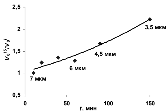
Рис. 2. Зависимость V_0^{15}/V_0^j от времени измельчения порошка для PbLα-линии
