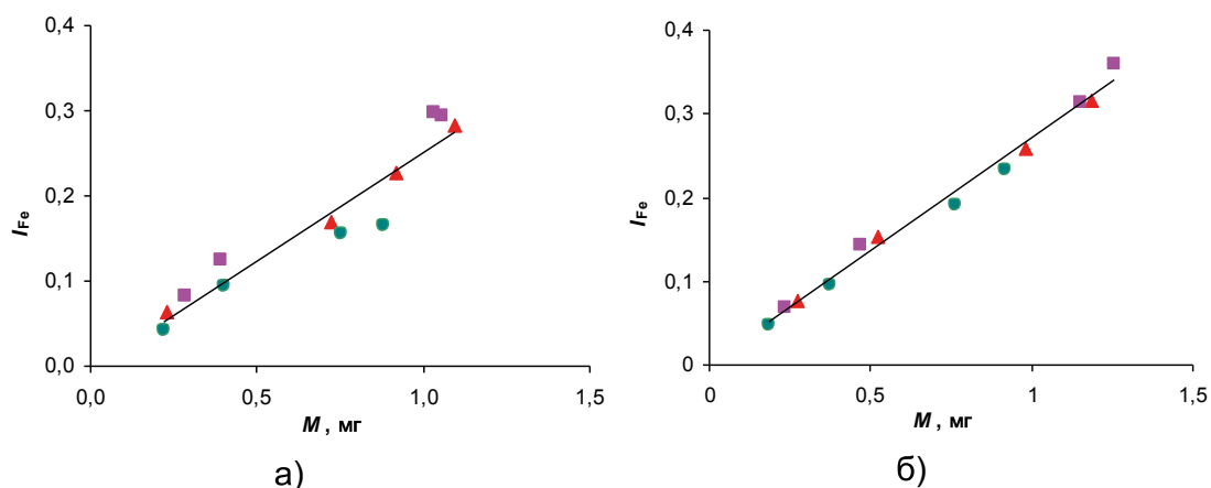
Рис. 1. Зависимость интенсивности FeKα-линии от массы Fe в излучателях Fe 3 O 4 (■), FeO (▲) и FeS 2 (●) при t (мин): а – 15, б – 150
