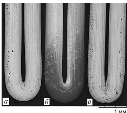
Рис. 3. Изображение кончиков зондов после: а – отжига-очистки, б – конденсации паров руды, в – конденсации паров палладия. Увеличение показано масштабным отрезком
