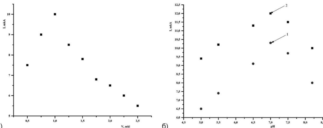
Рис. 3. а) Зависимость величины аналитического сигнала (ток окисления пероксида водорода) от количества ГО; б) Зависимость величины аналитического сигнала от pH буферных растворов для биосенсора два (кривая 1) и три (кривая 2) типов в системе фермент – субстрат – ингибитор MAO: MAO – дофамин – феназепам
