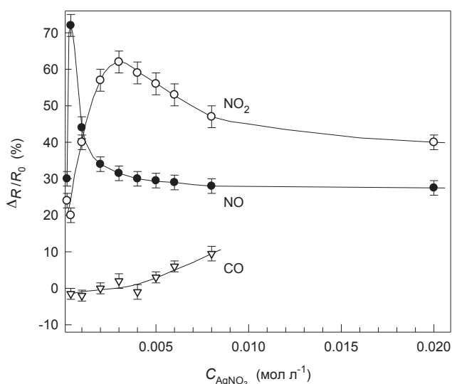
Рис 3. Отклик сенсорных элементов на основе пленок \text{Ag}_x\text{Pb}_{1-x}\text{S} , полученных из растворов с различной концентрацией нитрата серебра, после пятиминутного контакта с газовой смесью при температуре 295 К. Концентрация газа в смеси с воздухом: (○) 200\text{ мг}\cdot\text{м}^{-3} \text{NO}_2 , (●) 220\text{ мг}\cdot\text{м}^{-3} \text{NO} , (▽) 166\text{ мг}\cdot\text{м}^{-3} \text{CO}
