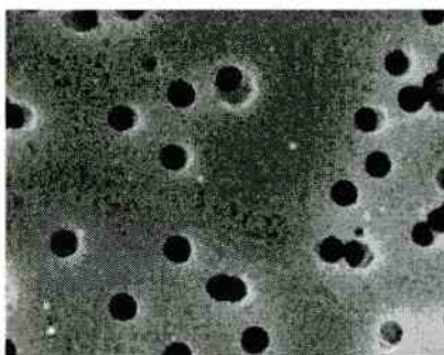
Рис. 2, в. Пример формирования трехмерного изображения поверхности полимерной трековой мембраны: 2-D изображение 38x30 мкм поверхности полимерной мембраны с порами 3 мкм и покрытием из TiN, время напыления 20 сек. РЭМ, увеличение 5000.
