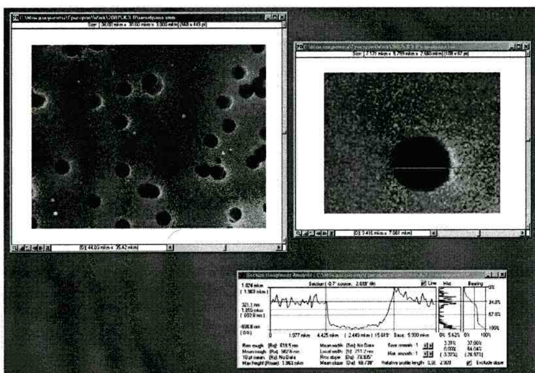
Рис. 2, г. Пример формирования трехмерного изображения поверхности полимерной трековой мембраны: показаны 2-D изображения размерами 38x30 мкм (РЭМ, рис. 2в) и 7.171x5.759 мкм поверхности полимерной мембраны с порами 3 мкм и покрытием из TiN. 2-D изображение размером 7.171x5.759 мкм поверхности получено путем копирования с увеличением фрагмента с порой из изображения 38x30 мкм. В нижней части рисунка показан профиль поверхности линии, проведенной через пору на 2-D изображении размером 7.171x5.759 мкм. Все изображения получены с помощью программы Scan Master.
