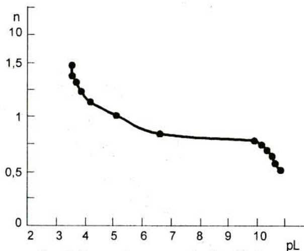
Рис.3. Кривая образования Zn : Nta = 1 : 2. C_{Zn} = 10^{-3} моль/л, C_L = 2 \cdot 10^{-3} моль/л
