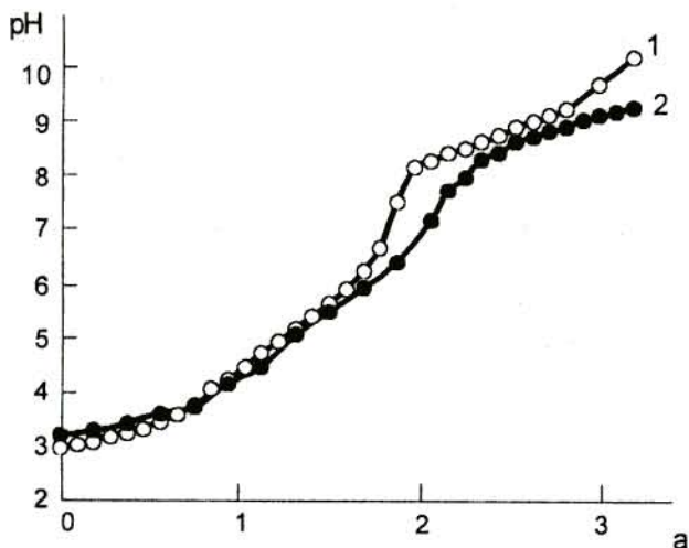
Рис.5. Кривые pH-потенциометрического титрования: 1 – Zn : Ida = 1 : 1, C_{Zn} = C_L = 2 \cdot 10^{-3} моль/л; 2 – Zn : Ida : Gly = 1 : 1 : 1, C = 10^{-3} моль/л
