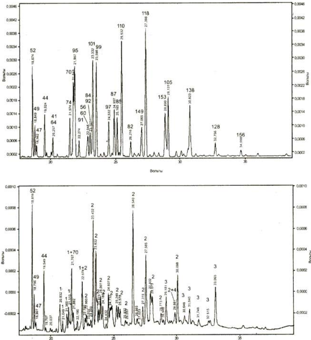
Рис. 1. Хроматограммы ГХ-ПИД: а) смеси ПХБ – Совол; б) продуктов реакции гидролиза ПХБ водным раствором гидроксида калия в диметилсульфоксиде: 1 – C_{12}H_6Cl_3OH ; 2 – C_{12}H_5Cl_4OH ; 3 – C_{12}H_4Cl_5OH ; 4 – C_{12}H_3Cl_6(OH)_2
