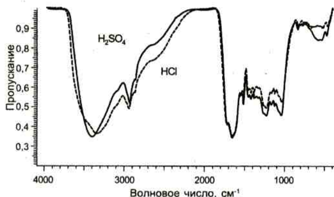
Рис.1. ИК спектры образцов 1 (HCl, прерывистая линия) и 2 (H 2 SO 4 , сплошная линия)
