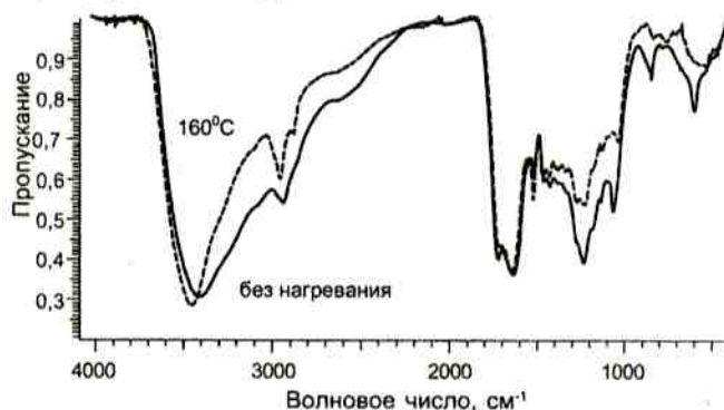
Рис.3. ИК спектры образцов 3 (без нагревания, сплошная линия) и 6 (160°C, прерывистая линия)
