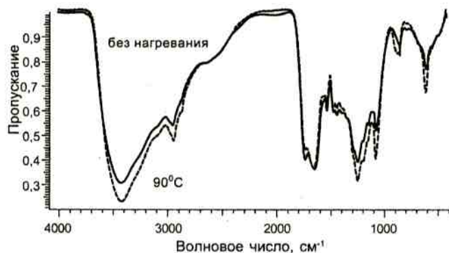
Рис.2. ИК спектры образцов 3 (без нагревания, сплошная линия) и 4 (90°C, прерывистая линия)
