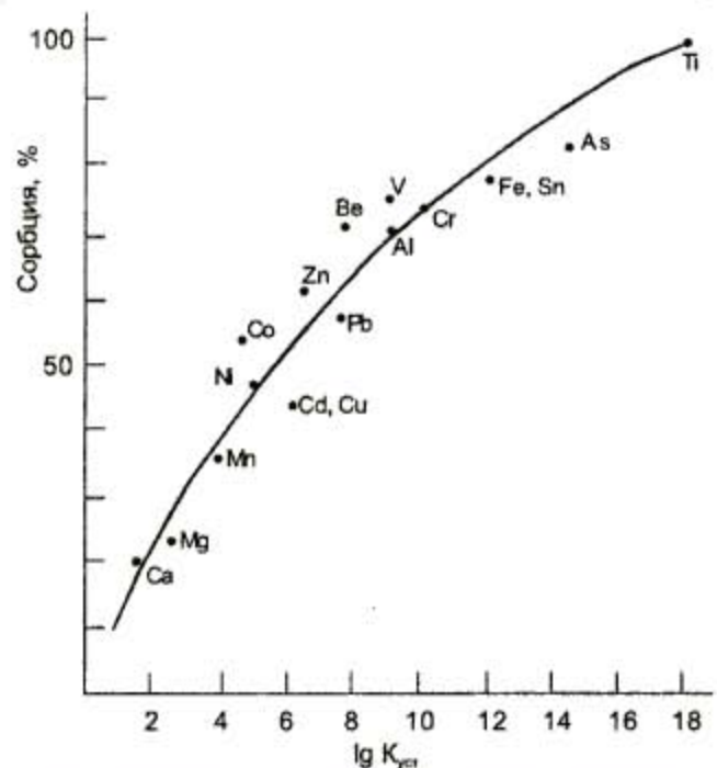
Рис. 2. Зависимость эффективности сорбции металлов от логарифмов константы устойчивости K_{уст.} их гидроксикомплексов ( \text{pH} = 7-8 )
