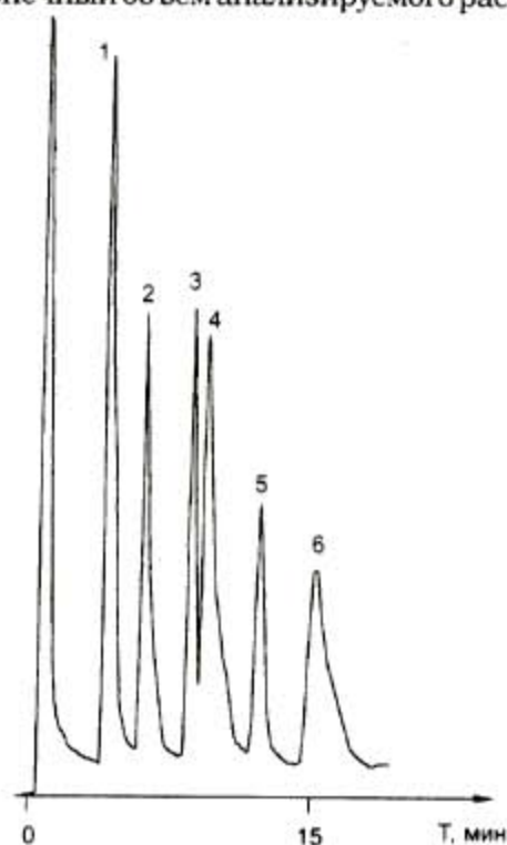
Рис.3. Хроматограмма раствора пентафторфенилгидразонов с концентрацией 1 мкг/мл (условия 2): 1 – ацетальдегида; 2 – пропаналя; 3 – метилэтилкетона; 4 – бутаналь; 5 – диэтилкетона; 6 – пентаналь
