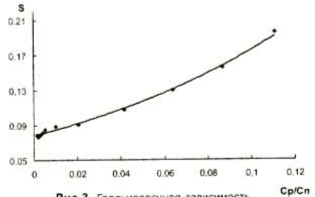
Рис.3. Градуировочная зависимость
