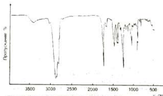
Рис.1. ИК спектр \text{CO}_2 -экстракта древесной зелени пихты сибирской (стрелкой указана полоса 860 \text{cm}^{-1} )
