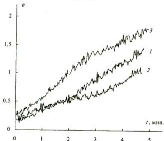
Рис. 7. Кривые зависимости термолинзового сигнала \vartheta от времени для окисления 1 \cdot 10^{-2} М анилина бромат-ионами ( 3 \cdot 10^{-2} М) в присутствии ванадия (V) ( 4 \cdot 10^{-2} М) в отсутствие 8-оксихинолина (кривая 1) и в его присутствии на уровне 1 \cdot 10^{-4} М (кривая 2) и 1 \cdot 10^{-3} М (кривая 3); \lambda_0 = 488,0 нм, мощность индуцирующего излучения 40 мВт
