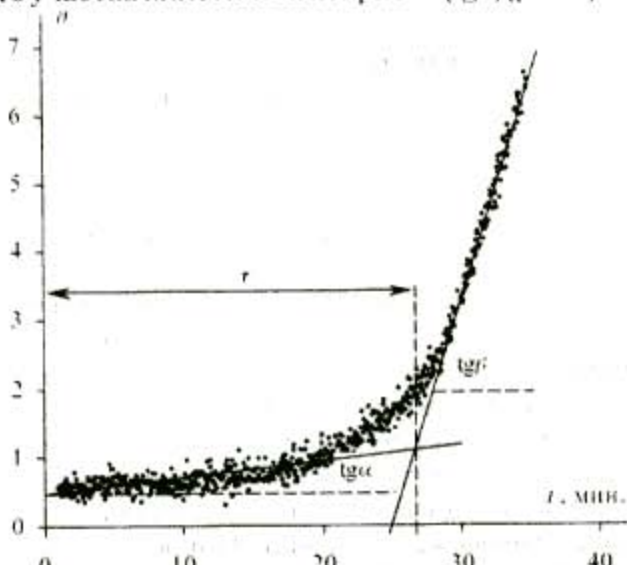
Рис.3. Зависимости термолинзового сигнала D от времени для окисления 1 \cdot 10^{-2} М анилина бромат-ионами ( 3 \cdot 10^{-2} М) в присутствии ванадия (V) ( 4 \cdot 10^{-7} М); \lambda_0 = 488,0 нм, мощность индуцирующего излучения 80 мВт
