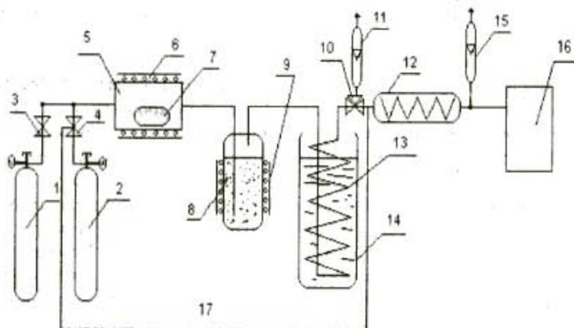
Установка для определения содержания водорода в металлах
