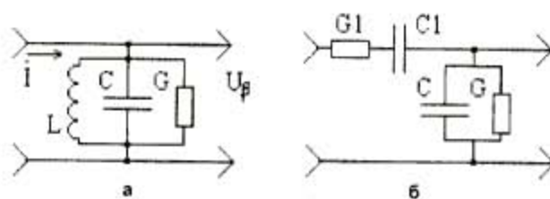
Рис.4. Цепи второго порядка, резонансная (а) и квазирезонансная (б), содержащие параллельные СG двухполюсники
