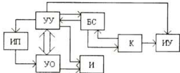
Рис.1. Функциональная схема диэлькометра
