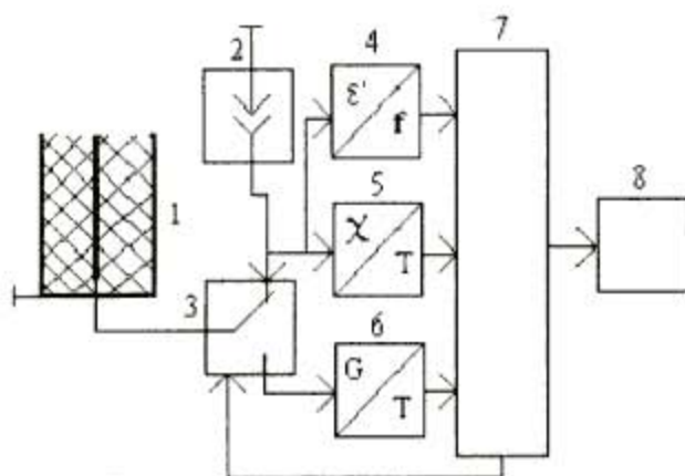
Рис.7. Многофункциональный дизелькометрический преобразователь
