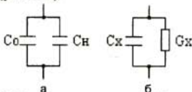
Рис.2. Эквивалентные схемы ПИП и образца
