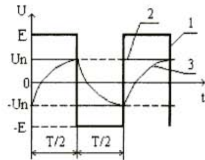
Рис. 6. Переходные процессы в базовом модуле: 1- форма импульсов в узле 1; 2 – форма импульсов в узле 2; 3 – форма импульсов в узле 3
