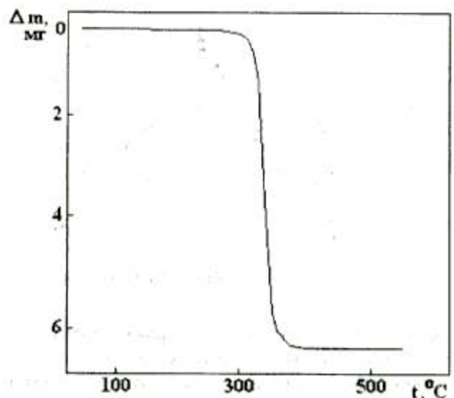
Рис. 2. Кривая ТГ механической смеси состава Ti_2O_3 + 4V_2O_5
