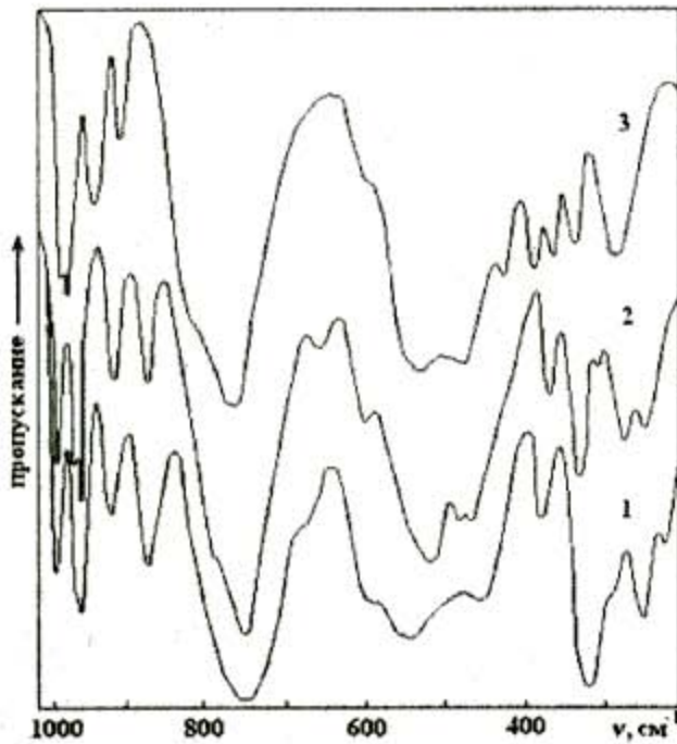
Рис.4. ИК спектры Ti_2V_8O_{21} (1), K_2V_8O_{21} (2), K_2V_8O_{20.8} (3)
