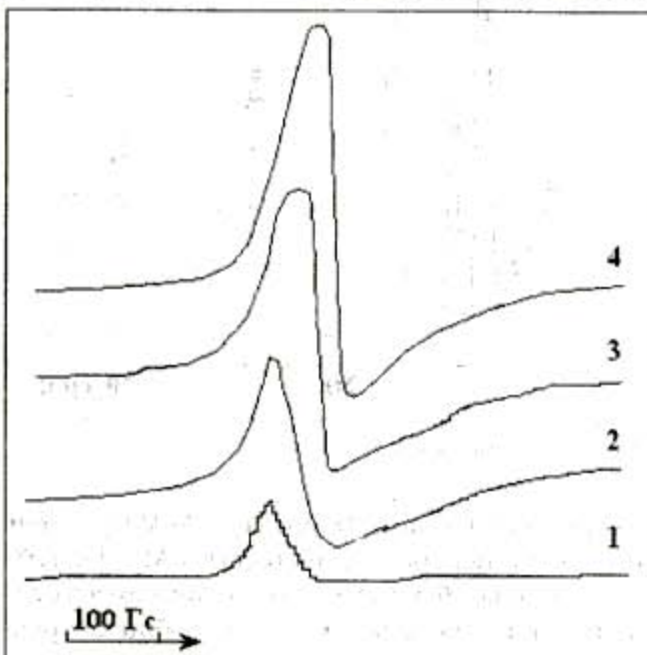
Рис. 1. Спектры ЭПР образца K_2V_8O_{21} , отожженного на воздухе при 475 (1), 500 (2), 525 (3), 550^\circ\text{C} (4)
