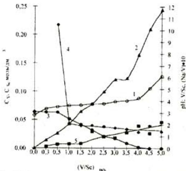
Рис.2. Зависимости значений pH растворов (1), молярных концентраций ванадия (2) и скандия (3) в растворах, мольных отношений V/Sc (4) и Na/V (5) в твердых фазах от исходного мольного отношения V/Sc при взаимодействии нитрата скандия с метаванадатом натрия в системе Sc(NO 3 ) 3 -Na 4 V 4 O 12 -H 2 O
