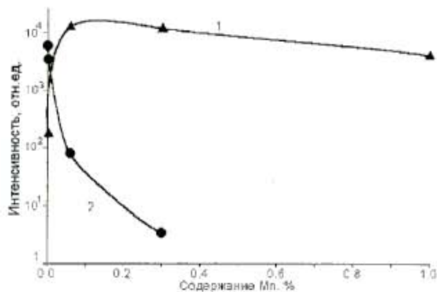
Рис.3. Зависимость интенсивностей внутрицентровой (1) и краевой (2) полос ИКЛ от содержания марганца в кристаллах ZnSe:Mn.
