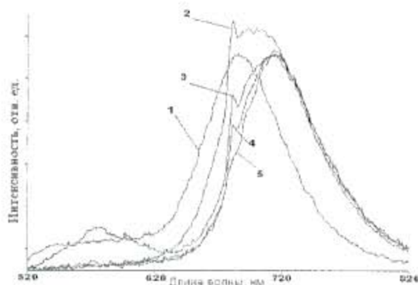
Рис.5. Спектр ИКЛ разновидностей берилла (режим «А»): бесцветный (1), прозрачный зеленоватый (2), непрозрачный зеленый (3), в «рубашке» изумруда (4), изумруд (5).
