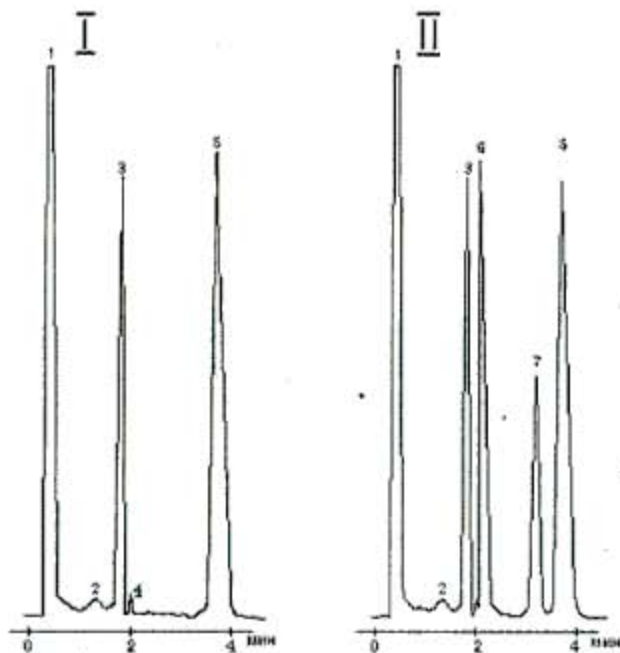
Рис.1. Хроматограммы раствора смеси камфоры и бромкамфоры (I) и этого же раствора с добавкой нафталина и дифенила (II). 1 - растворитель, 2,4 - неидентифицированные примеси, 3 - камфора, 5 - бромкамфора, 6 - нафталин, 7 - дифенил
