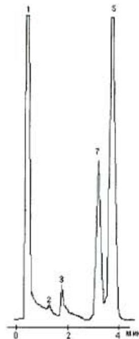
Рис.2. Характерная хроматограмма, полученная при определении примеси камфоры в бромкамфоре 1 - растворитель, 2,4 - неидентифицированные примеси, 3 - камфора, 5 - бромкамфора, 6 - нафталин, 7 - дифенил
