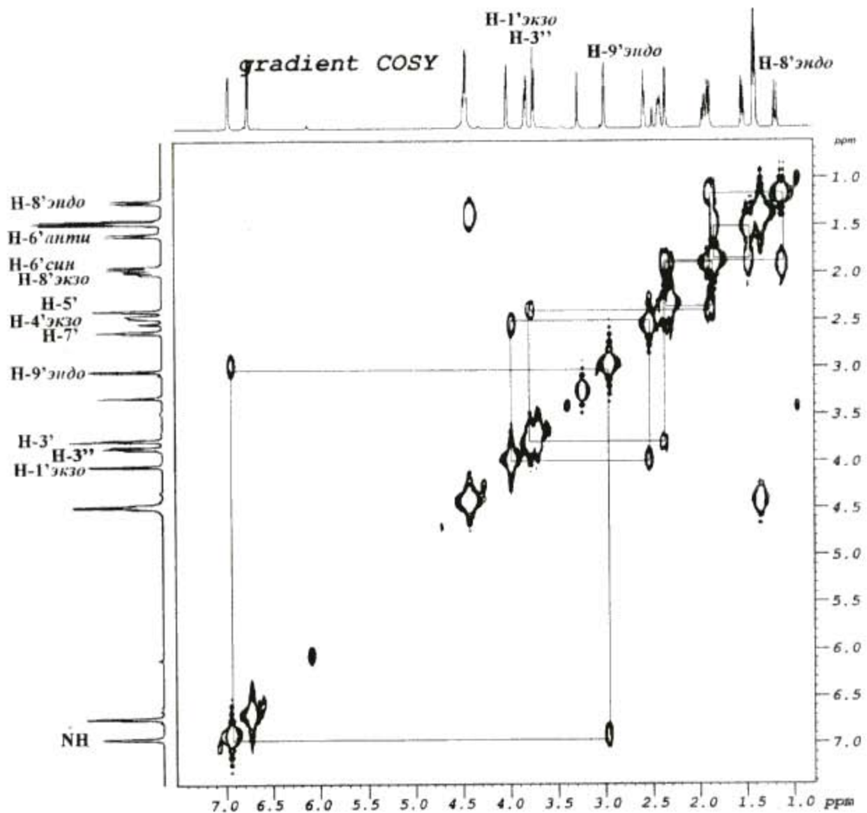
Рис.3. Двумерный 1 H- 1 H корреляционный ЯМР спектр (COSY) соединения 9.
