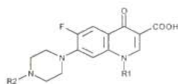
Схема 1. Структура некоторых антибактериальных препаратов фторхинолонового ряда (в скобках приведены торговые названия).
