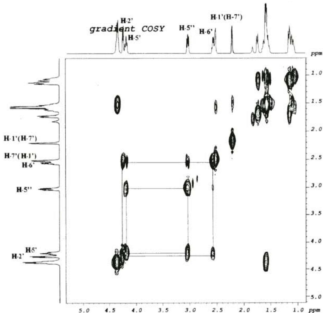
Рис 7. Двумерный ^1\text{H} - ^1\text{H} корреляционный спектр соединения II.
