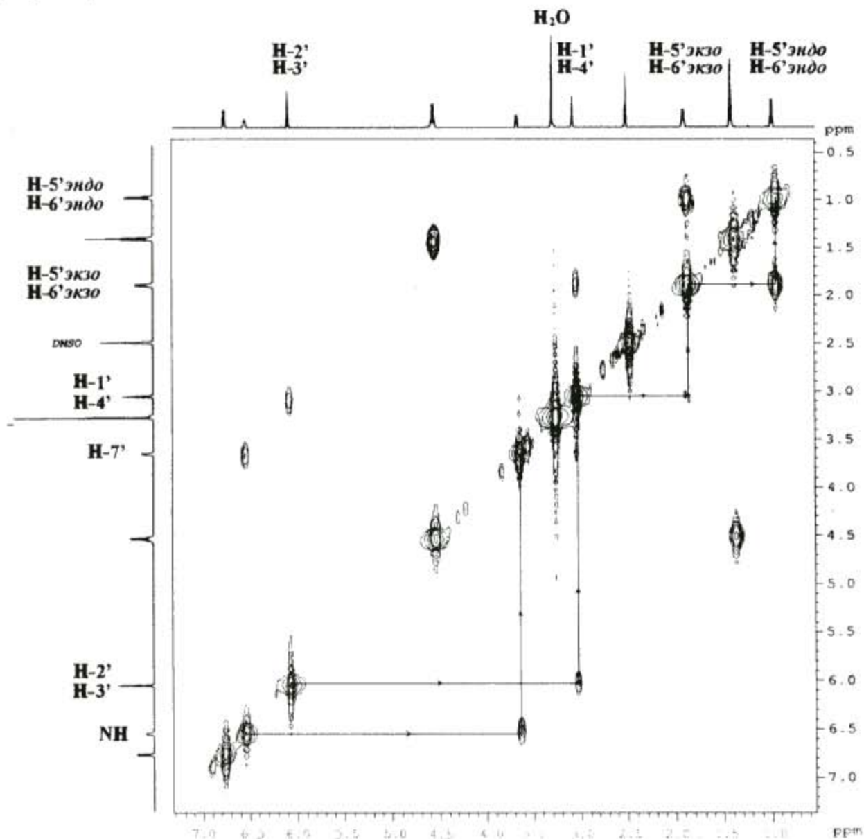
Рис.1. Двумерный ^1\text{H} - ^1\text{H} корреляционный ЯМР спектр (COSY) соединения 8 .
